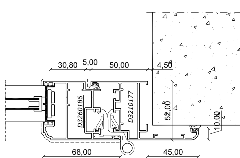
Sezione B - orizzontale
