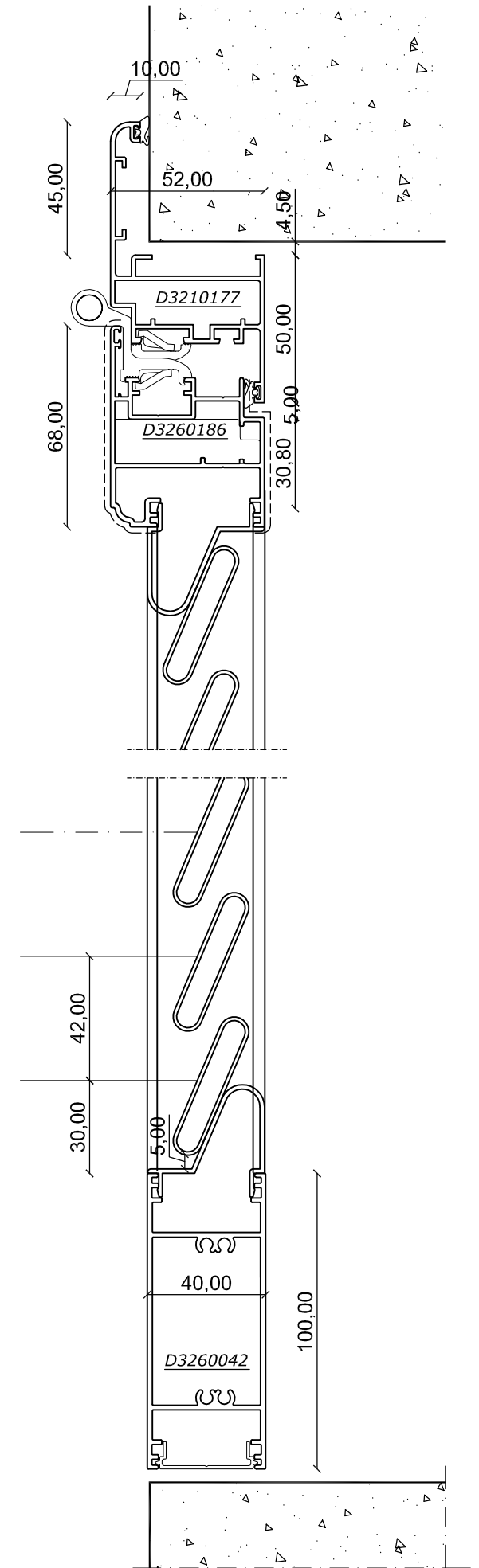
Sezione A - verticale
