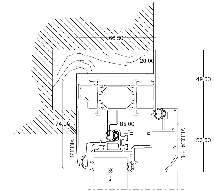
Sezione A - verticale
